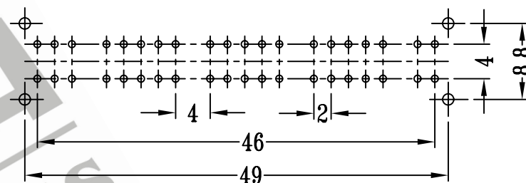
P.C.B LAYOUT
